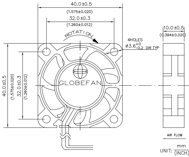
外形圖 外形図 Outline
