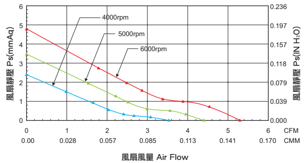
風量, 靜壓特性曲線 風量, 静圧特性カーブ Characteristic Curves
