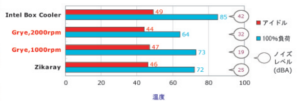
CPU温度 ノイズレベル比較表 100%負荷時 / アイドル時（周辺温度35℃）
